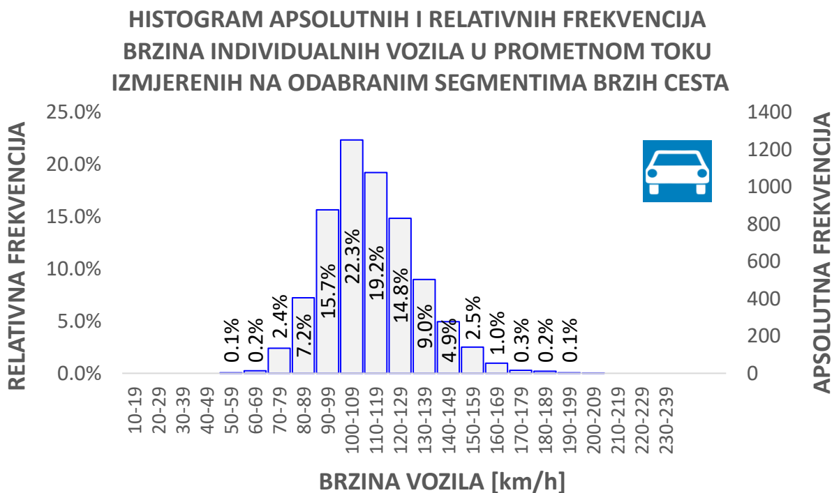
Grafikon 9. Empirijska razdioba apsolutnih i relativnih učestalosti (frekvencija) izmjerenih vrijednosti brzine individualnih vozila u prometnom toku na odabranim segmentima brzih cesta u Republici Hrvatskoj po definiranim statističkim razredima. Izvor: obrada autora.
