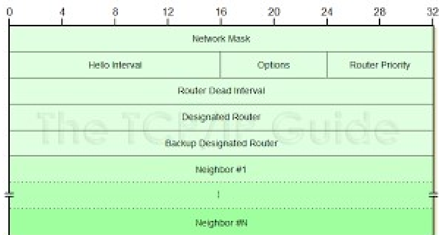
Slika 11. Hello paket [30]
