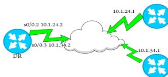
Slika 20. NBMA mreža [45]
