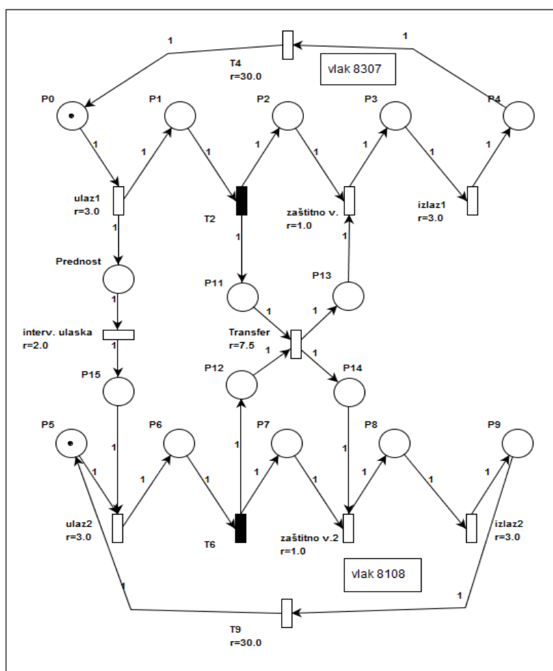
Slika 6.7: Petrijeva mreža jednog para vlakova
