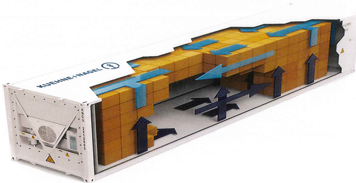
Slika 3 : Reefer kontejner
