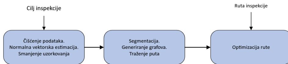
Slika 20. Prikaz procesa generiranja rute.
