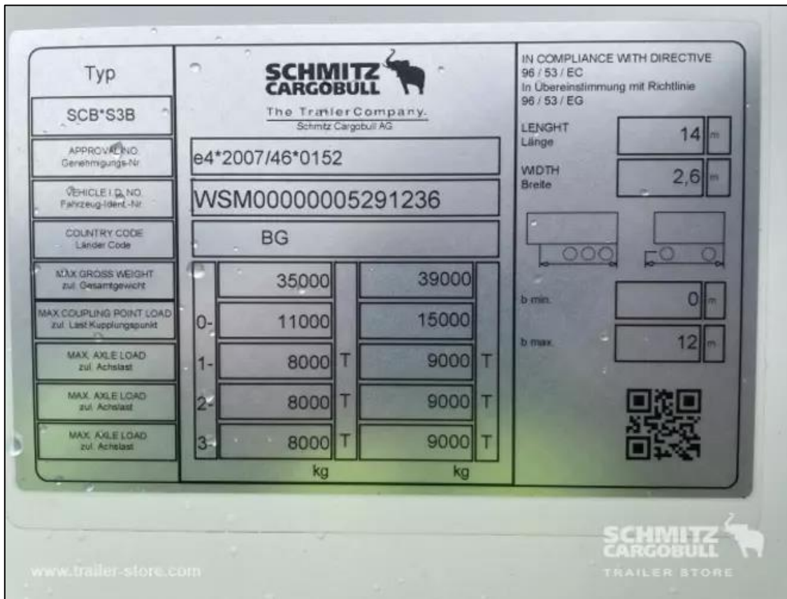
Slika 35. Eksploatacijske značajke troosovinske poluprikolice s temperaturnim režimom rada SCHMITZ proizvođača marke FERROPLAST koje su postavljene na prednjoj strani poluprikolice,
