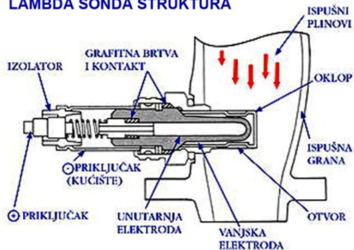
Slika 7 strukturni prikaz lambda sonde, [23]
