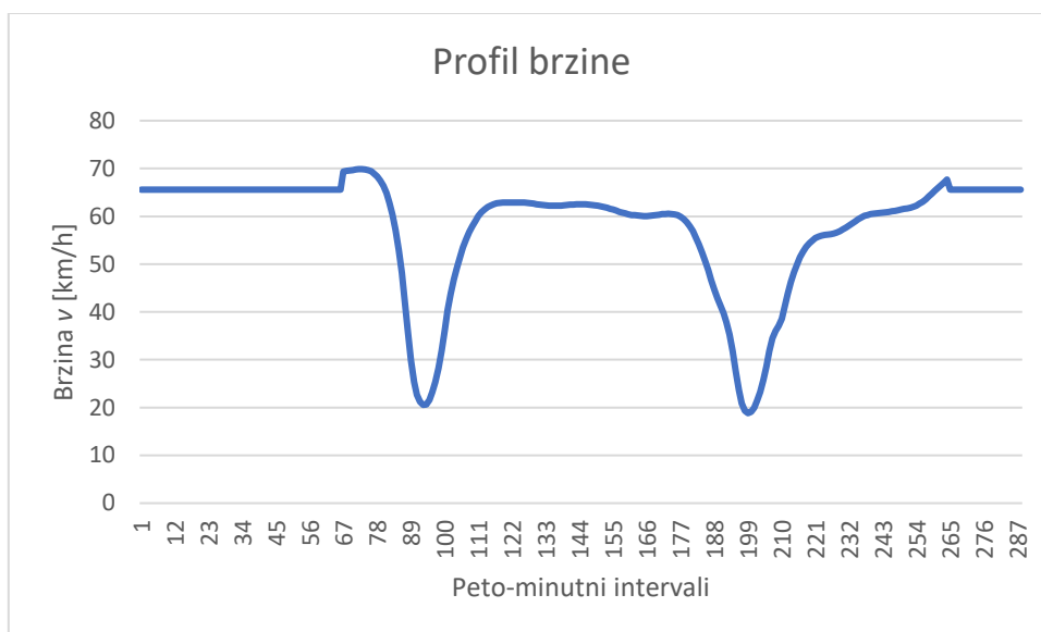
Slika 11. Profil brzine na Jadranskom mostu
