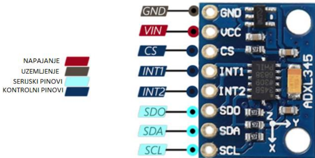
Slika 5 Akcelerometar ADXL345, [3]
