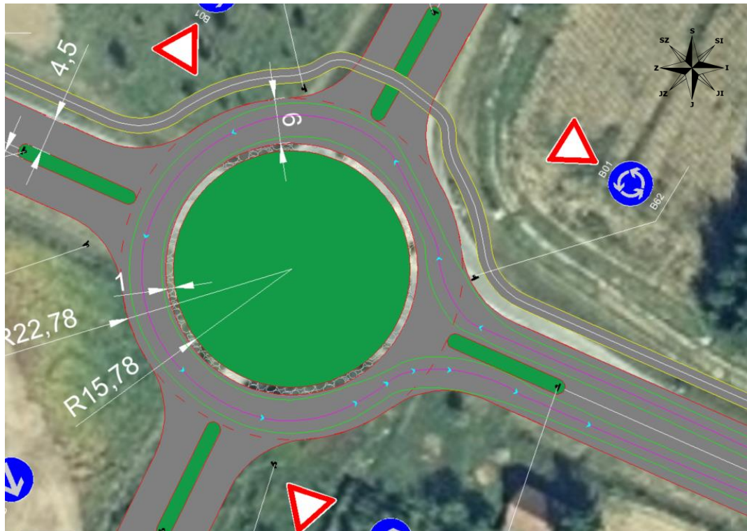
Slika 30.: Prikaz trajektorije vozila
