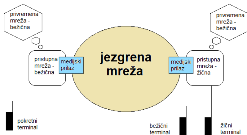
Slika 1. Arhitektura mreže,
