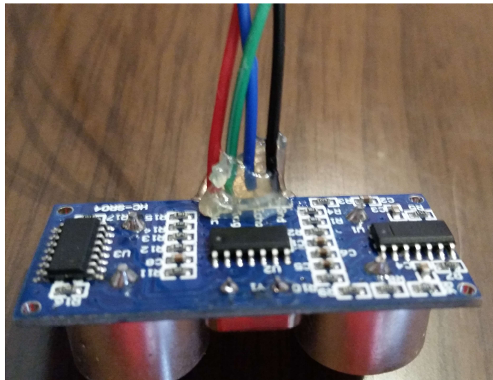
Slika 19 Zalemljeni vodiči ojačani vrućim ljevilom
