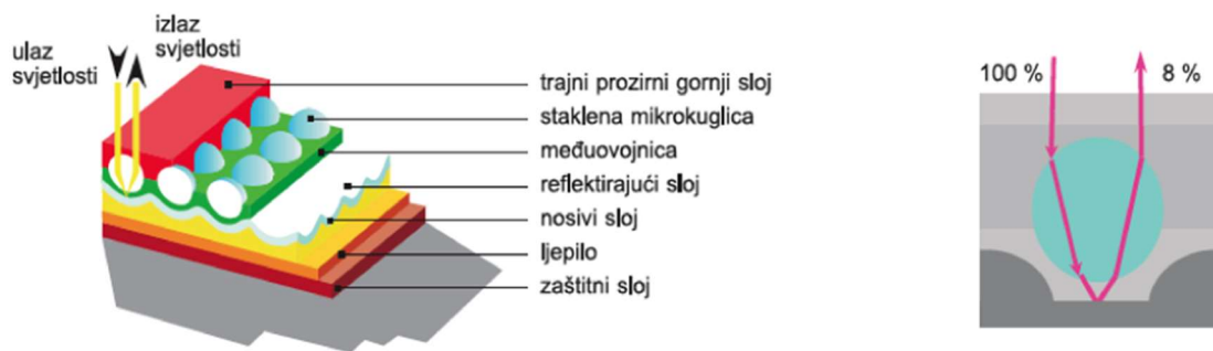
Slika 17. Retroreflektirajući materijal klase I
