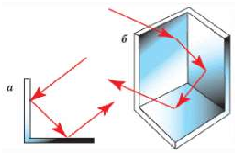
Slika 16. Prizmatična retrorefleksija
