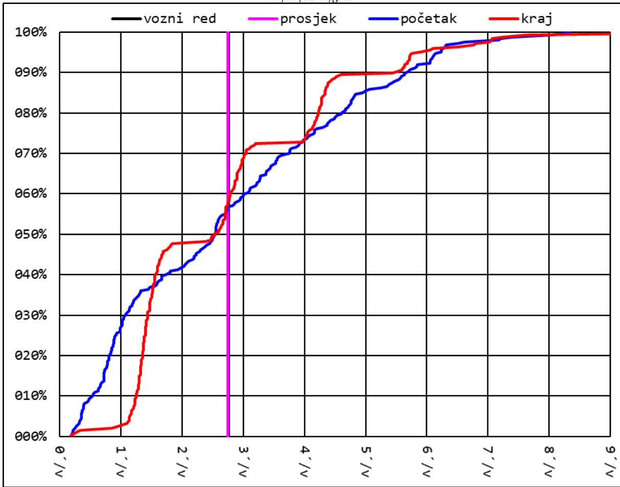
Prilog 36. Kumulativna razdioba sljedova vozila i kumulativni odnos krajnjeg i početnog slijeda, segment 06|30|vdkn|glk1
