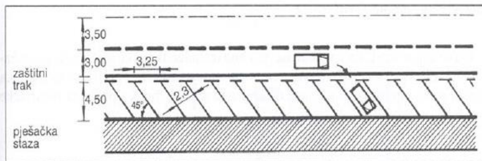
Slika 3. Koso parkiranje [5]
