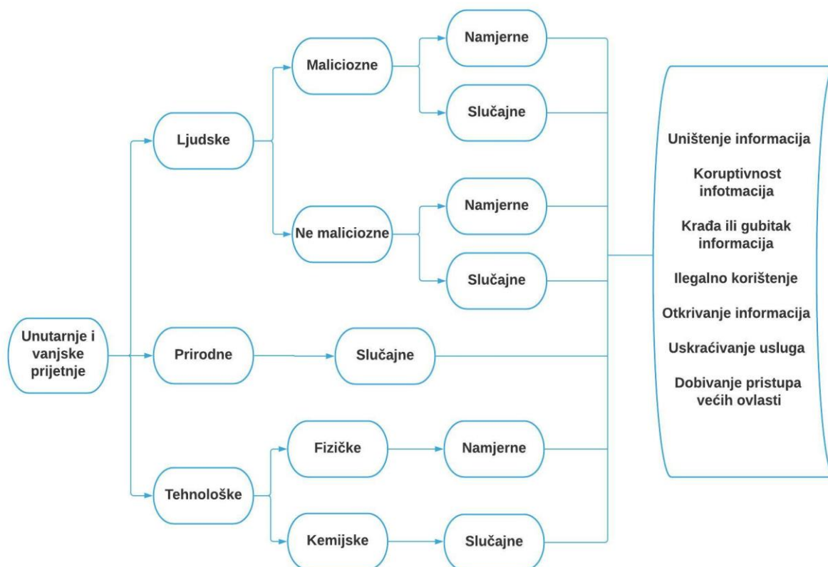
Slika 4. Klasifikacija prijetnji
