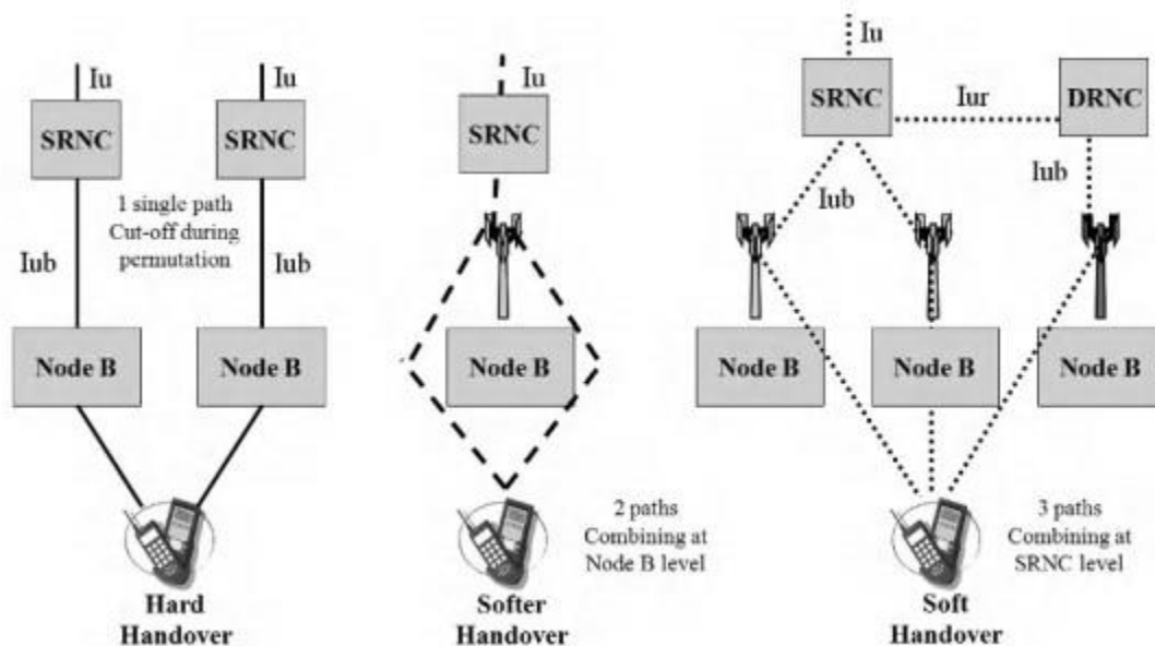
Slika 6. UMTS handover [1]
