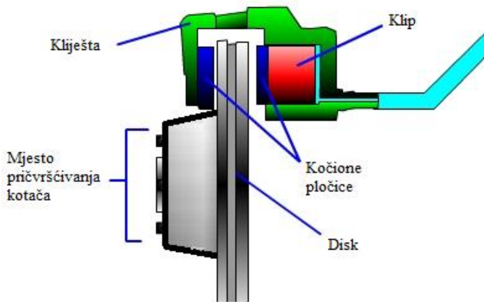
Slika 9. Disk kočnica
