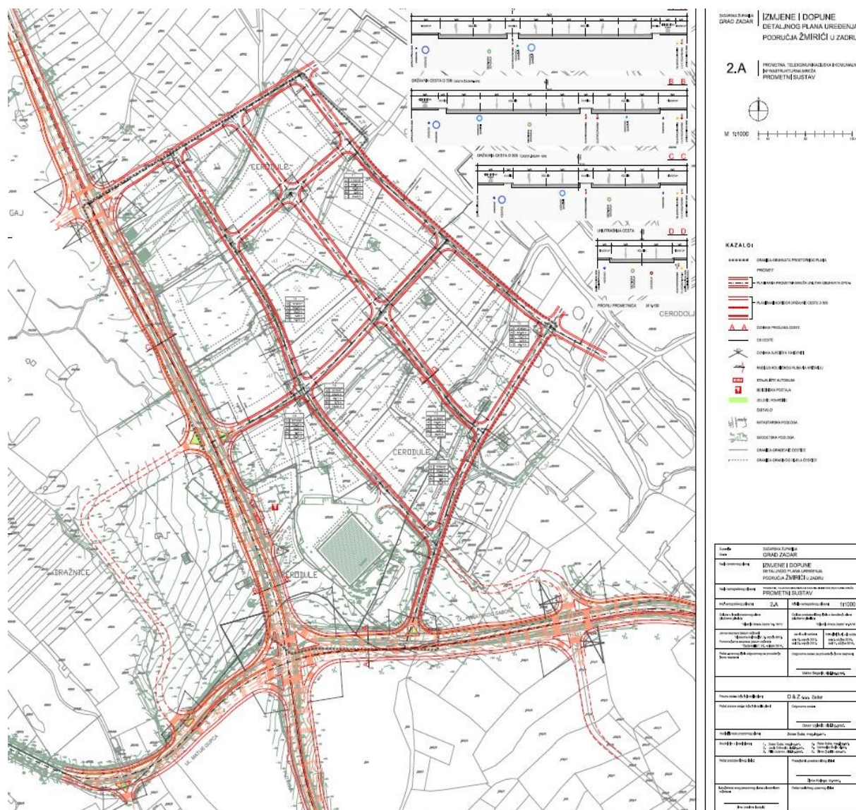
Slika 3.5. Detaljni plan uređenja područja „Žmiriči“ u Zadru
