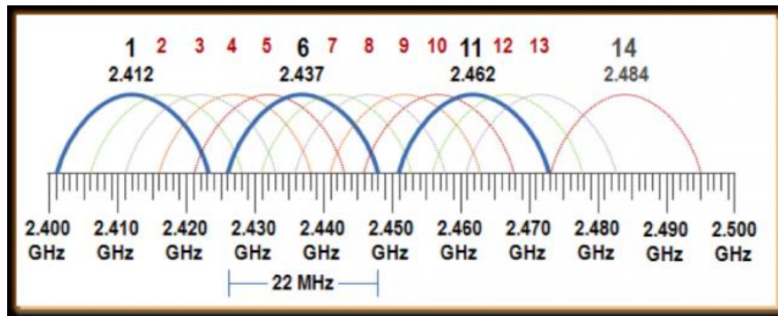
Slika 3. Plan iskoristivosti kanala frekvencijskog pojasa od 2.4 GHz, [27]
