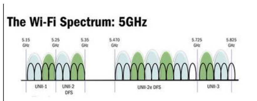
Slika 4. Plan iskoristivosti kanala frekvencijskog pojasa od 5 GHz, [29]
