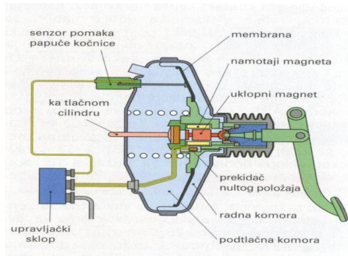
Slika 15. Komponente BAS-a [10]
