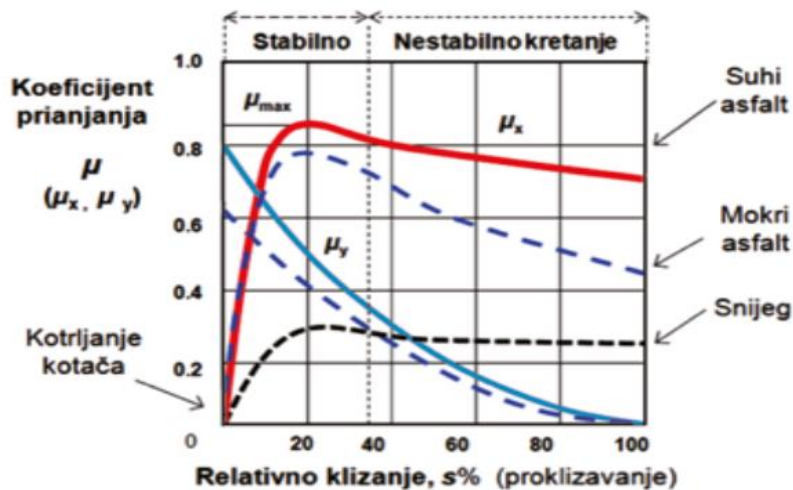
Slika 6. Dijagram koeficijenta prianjanja [5]
