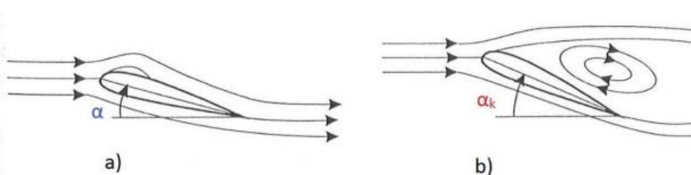
Slika 12. Mjehurasta zona odvajanja kod tankih aeroprofila s malim radijusom zakrivljenja nosa, a) umjeren napadni kut \alpha < \alpha_k , b) slom uzgona \alpha \geq \alpha_k
