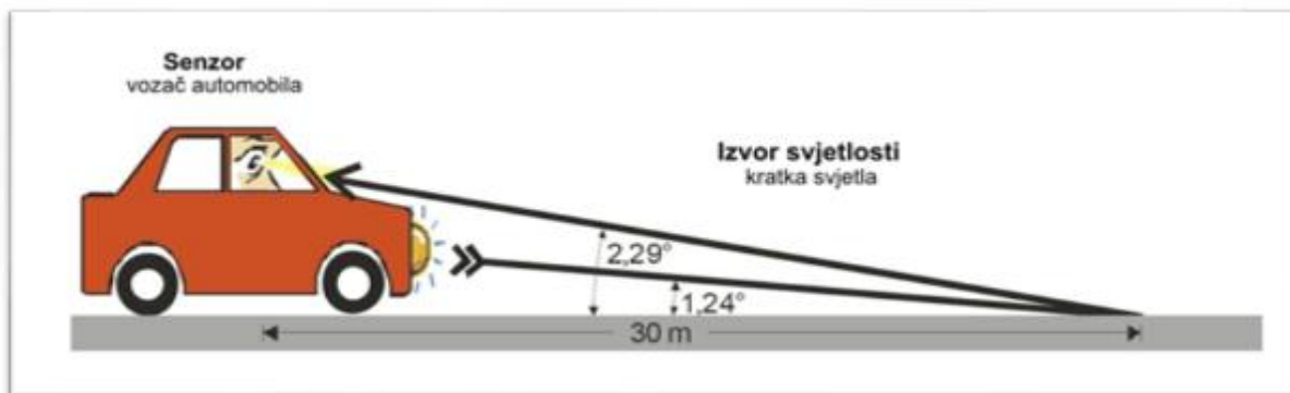
Slika 17. Princip mjerenja noćne vidljivosti
