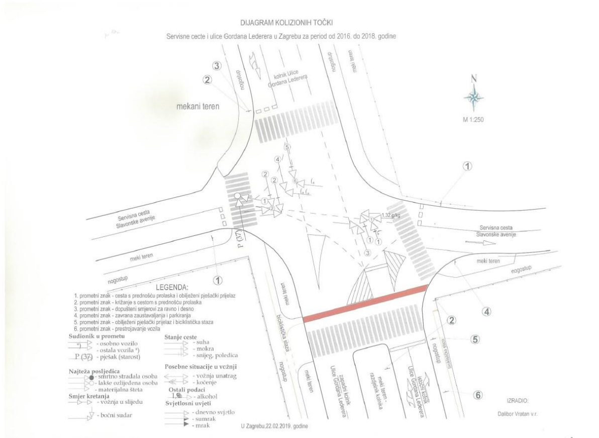
Slika 25 Dijagram kolizionih točaka
