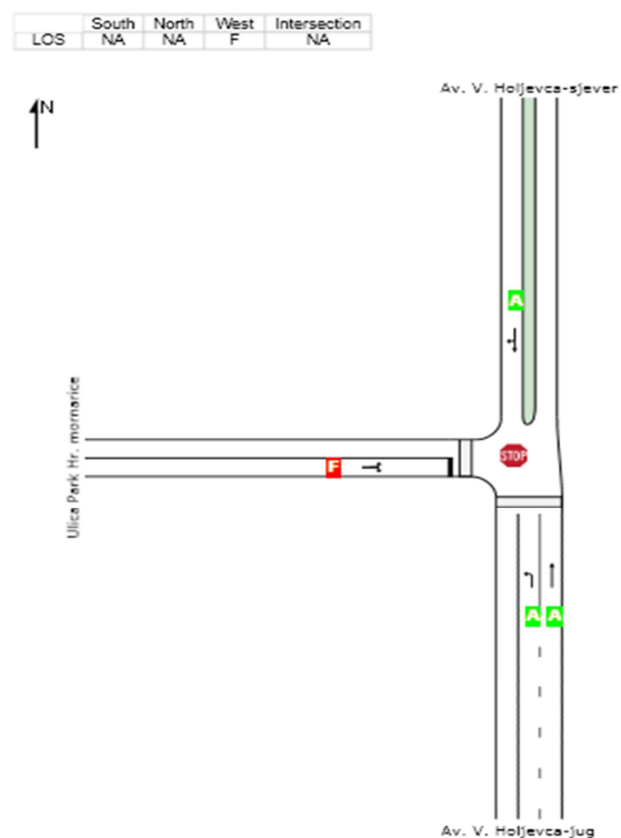
Slika 7. Analiza prometnih tokova uporabom simulacijskog alata SIDRA
