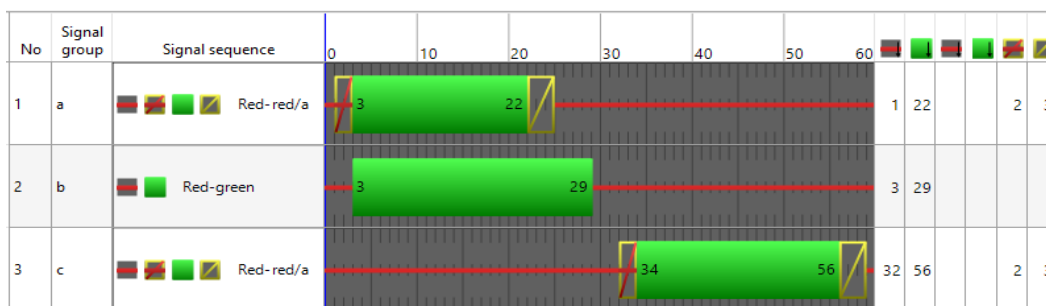
Slika 79.: Varijanta 4 - signalni plan
