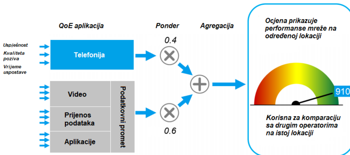
Slika 10. Ponderiranje i agregacija za geografsko područje
