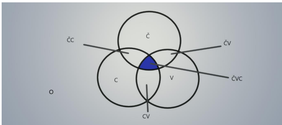
Slika 1. Vennov dijagram
