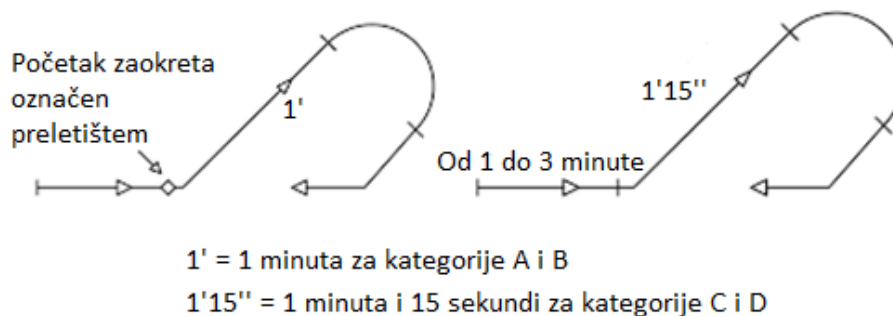
Slika 4. Proceduralni zaokret 45°/180°
