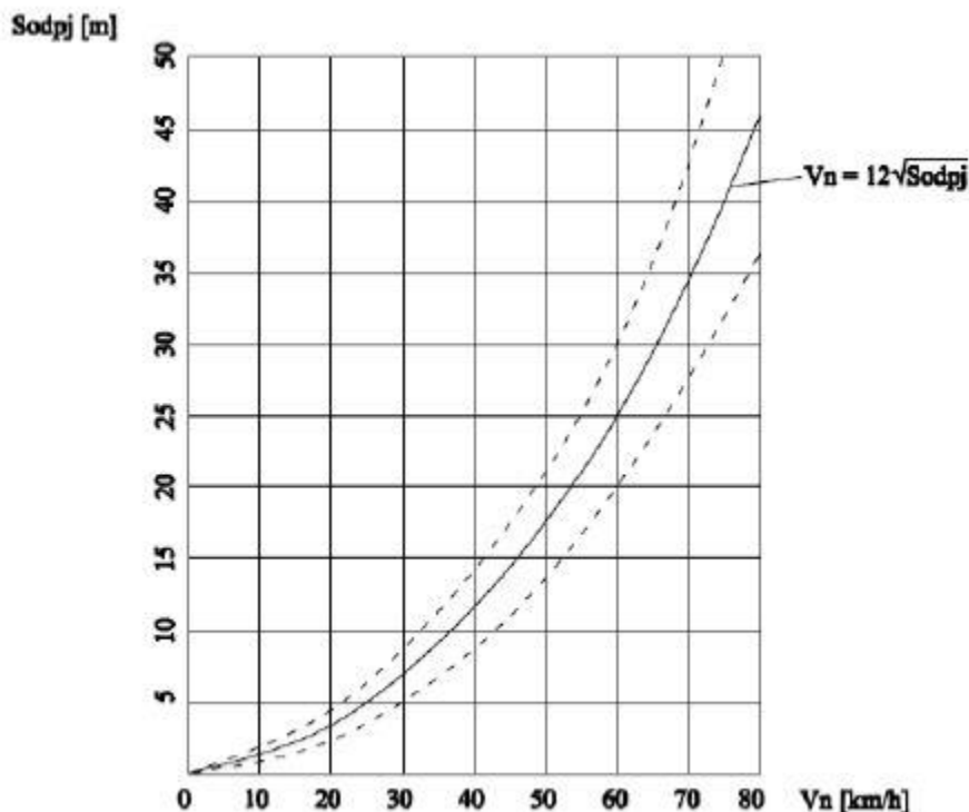
Slika 9. Dijagram daljine odbačaja pješaka u ovisnosti o naletnoj brzini vozila i intenzitetu kočenja [1]
