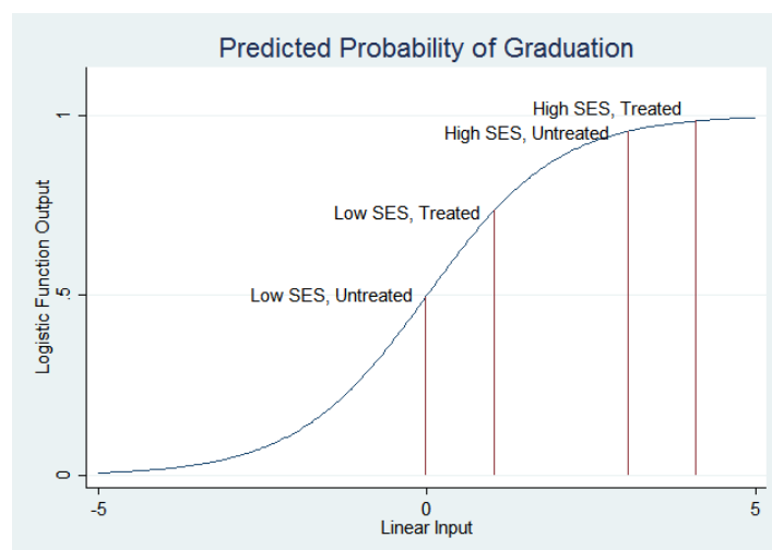
Slika 2. Primjer kontinuirane varijable, [3]
