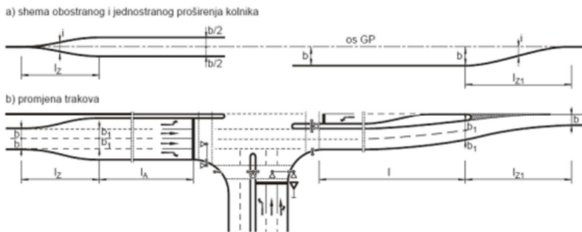
Slika 15. Promjena broja trakova na prilazu i izlazu s raskrižja, [4]
