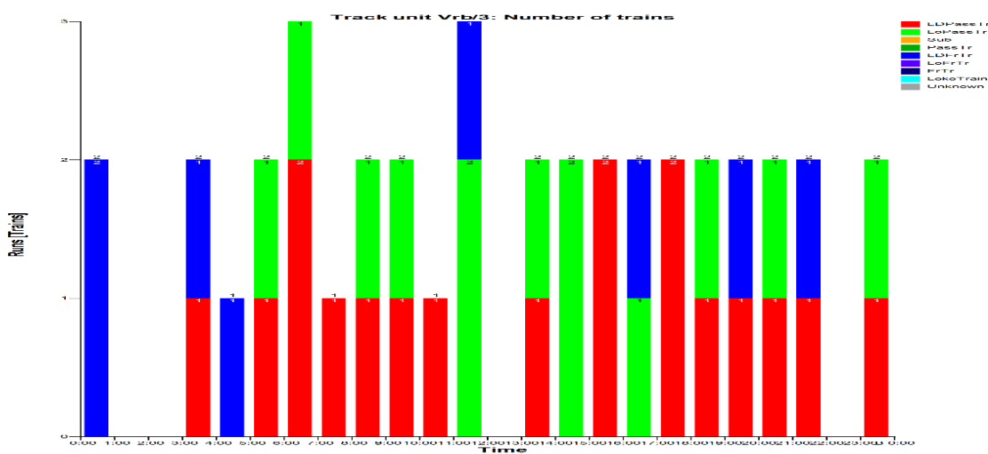
Grafikon 6. Zauzetost trećeg kolosijeka kolodvora Vrbovec
