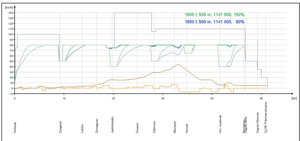
Grafikon 3.5. Ovisnost brzine vožnje o prijedenoj putu za teretni vlak na dionici Karlovac –Zagreb RK pri prolazu kolodvora vožnjom u pravac i vožnjom u skretanje
