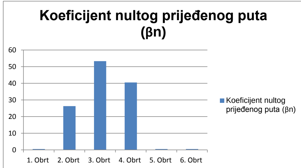
Grafikon 3. Prikaz koeficijenata nultog prijeđenog puta po pojedinim obrtima
