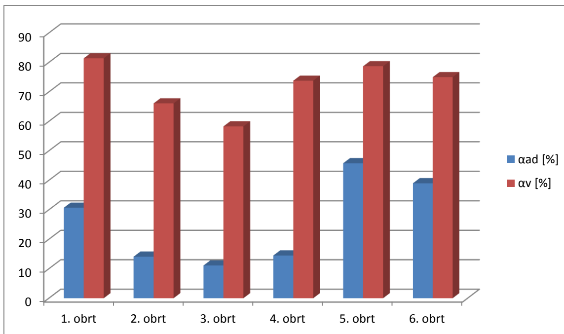
Grafikon 2. Prikaz koeficijenta angažiranosti i koeficijenta iskorštenja vozila u radu
