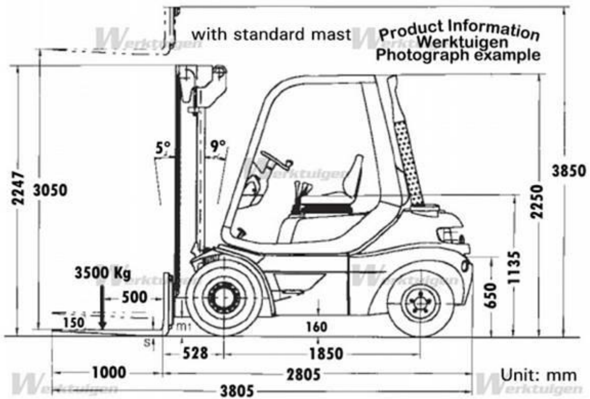
Slika 3: Gabariti i nosivost viličara Linde H35D, [8]
