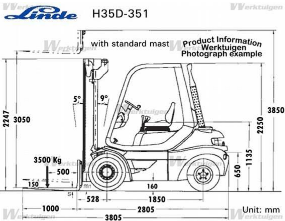
Slika 3: Gabariti i nosivost viličara Linde H35D, [8]
