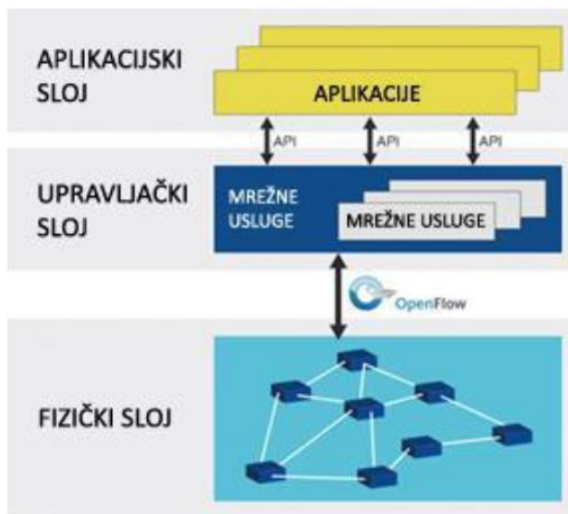
Slika 8. Arhitektura softverski definirane mreže, [17]
