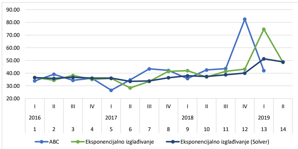
Grafikon 14 Grafički prikaz potražnje i prognoza potražnje (metoda eksponencijalnog izглаđivanja) za grupu proizvoda ABC (ADR)
