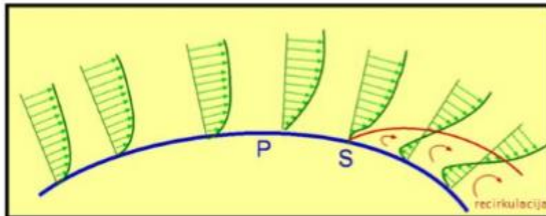
Slika 23. Odvajanje strujnica u točki S [7]
