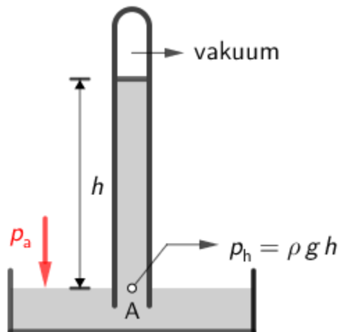
Slika 3. Mjerenje tlaka [3]
