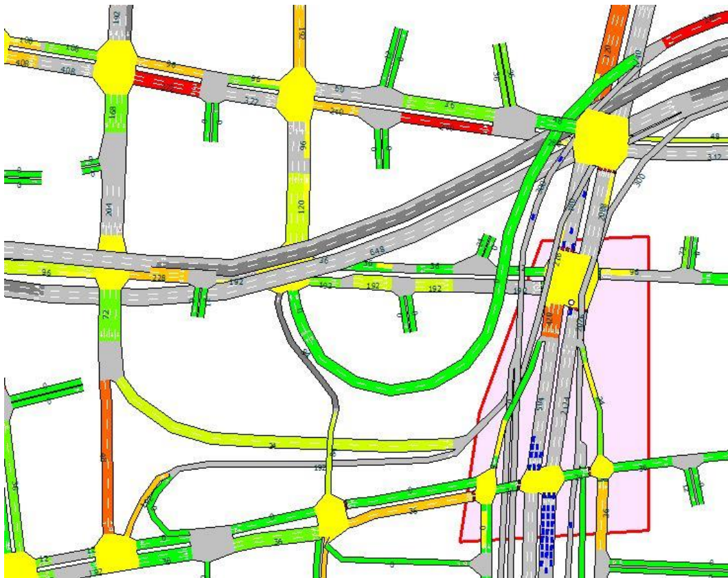
Slika 4. Mezoskopski model [4]
