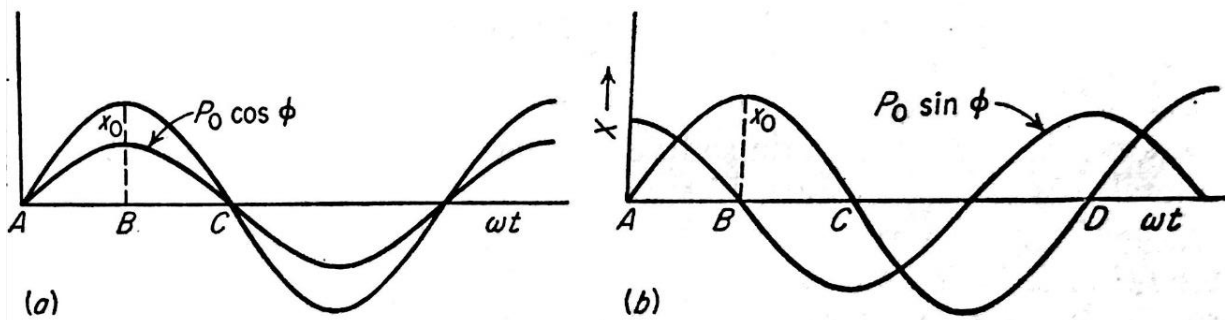
Slika 5. Dijagram komponenta sile sa harmonijskim gibanjem, [6]
