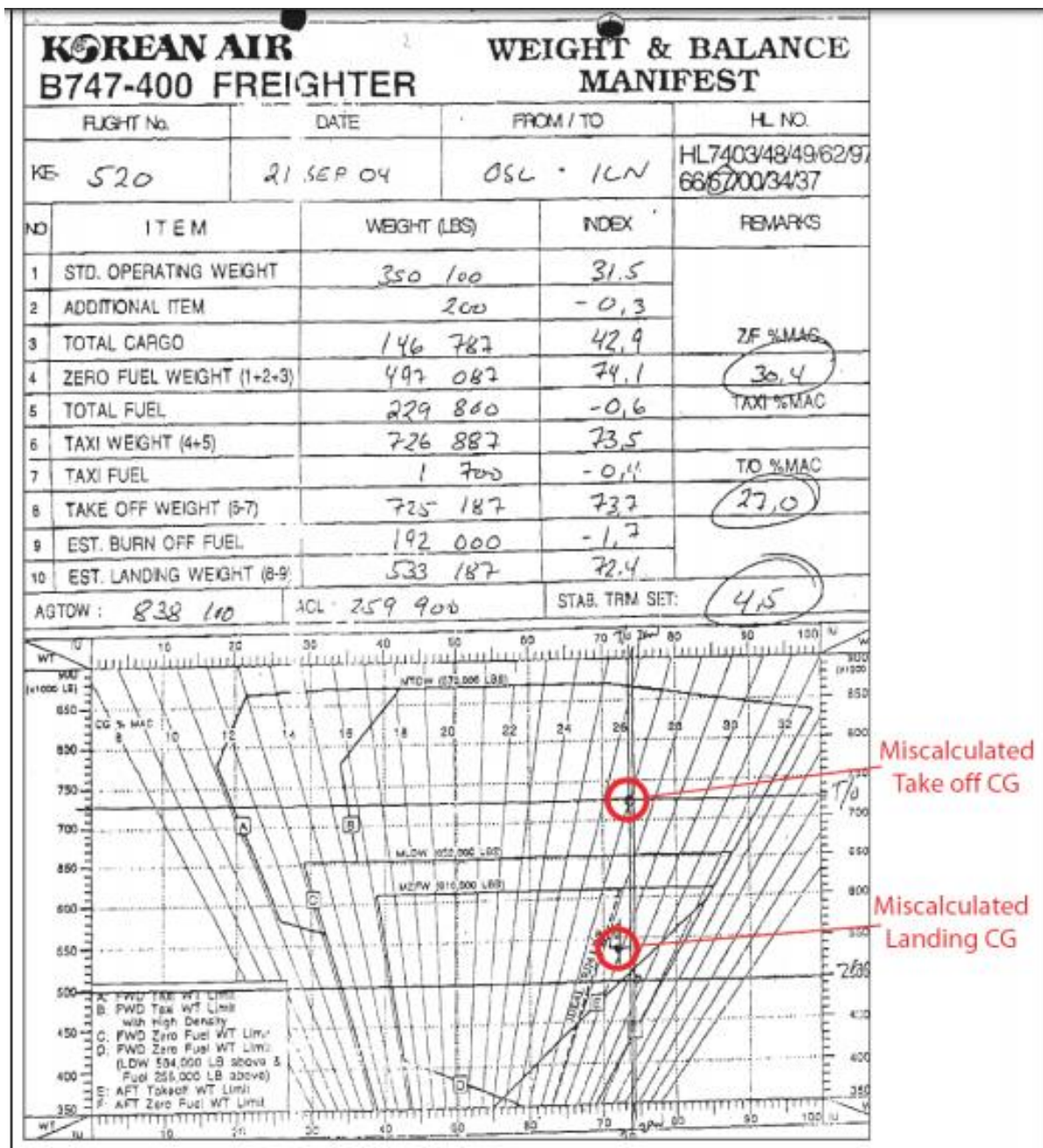
Slika 12. Pogrešna lista uravnoteženja i opterećenja zrakoplova Izvor: [19]
