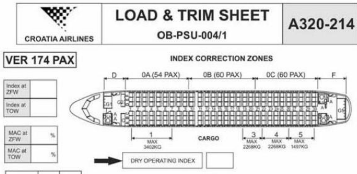
Slika 19. Zone indeksnih korekcija Izvor: [12]
