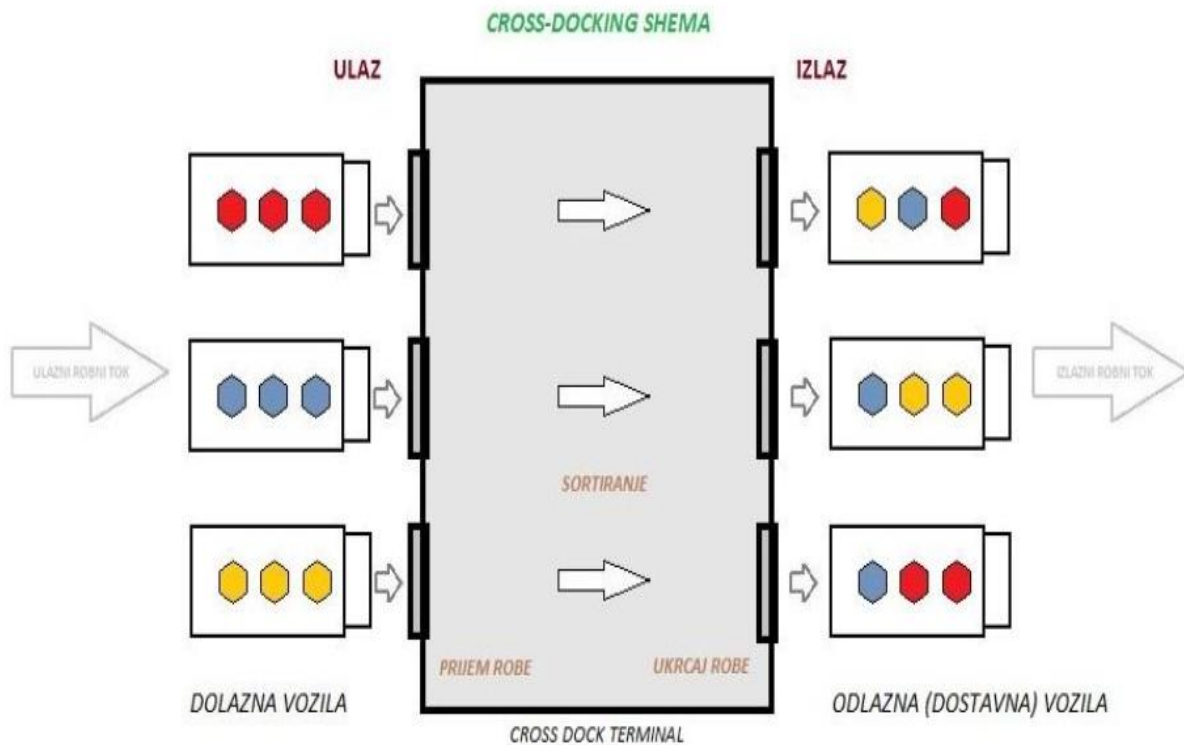
Slika 2. Sustav cross docking-a
