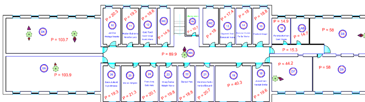
Slika 69 Raspoored pristupnih točaka na katu.
