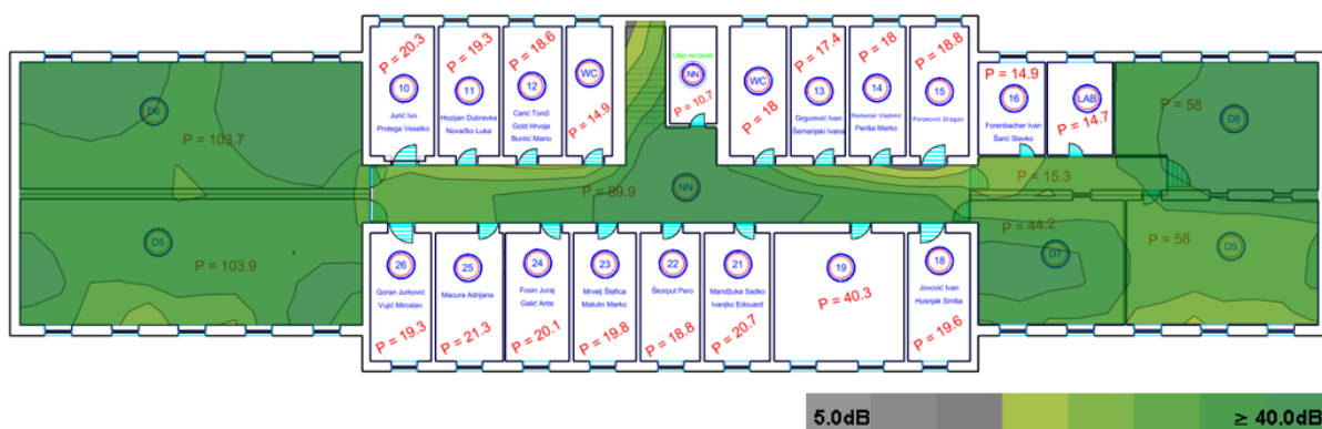
Slika 143 Omjer signal - šum u 5 GHz pojasu na katu.
