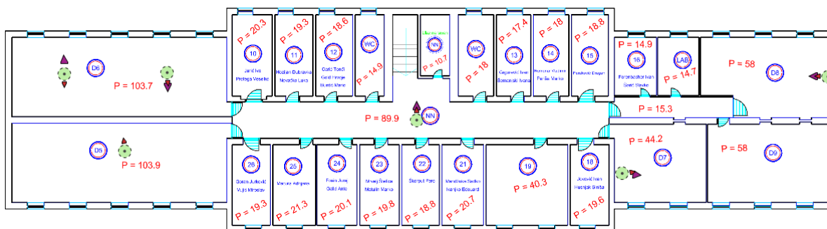
Slika 109 Raspoored pristupnih točaka na katu.
