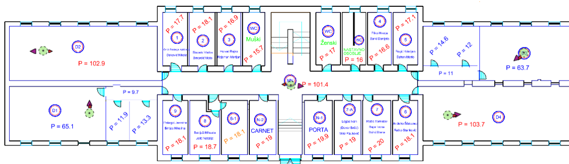
Slika 68 Raspoored pristupnih točaka u prizemlju.
