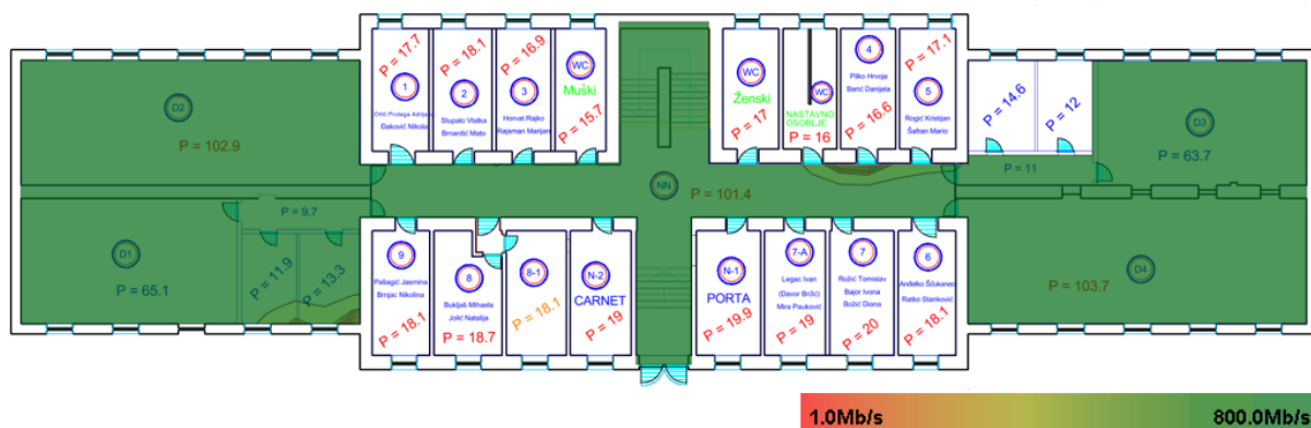
Slika 164 Brzina prijema u prizemlju u 5 GHz pojasu.
