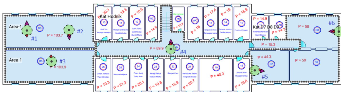
Slika 75 Prikaz pristupnih točaka na katu te usmjerenja njihovih antena, pri čemu manja strelica označava 5 GHz, a veća 2.4 GHz pojao.
