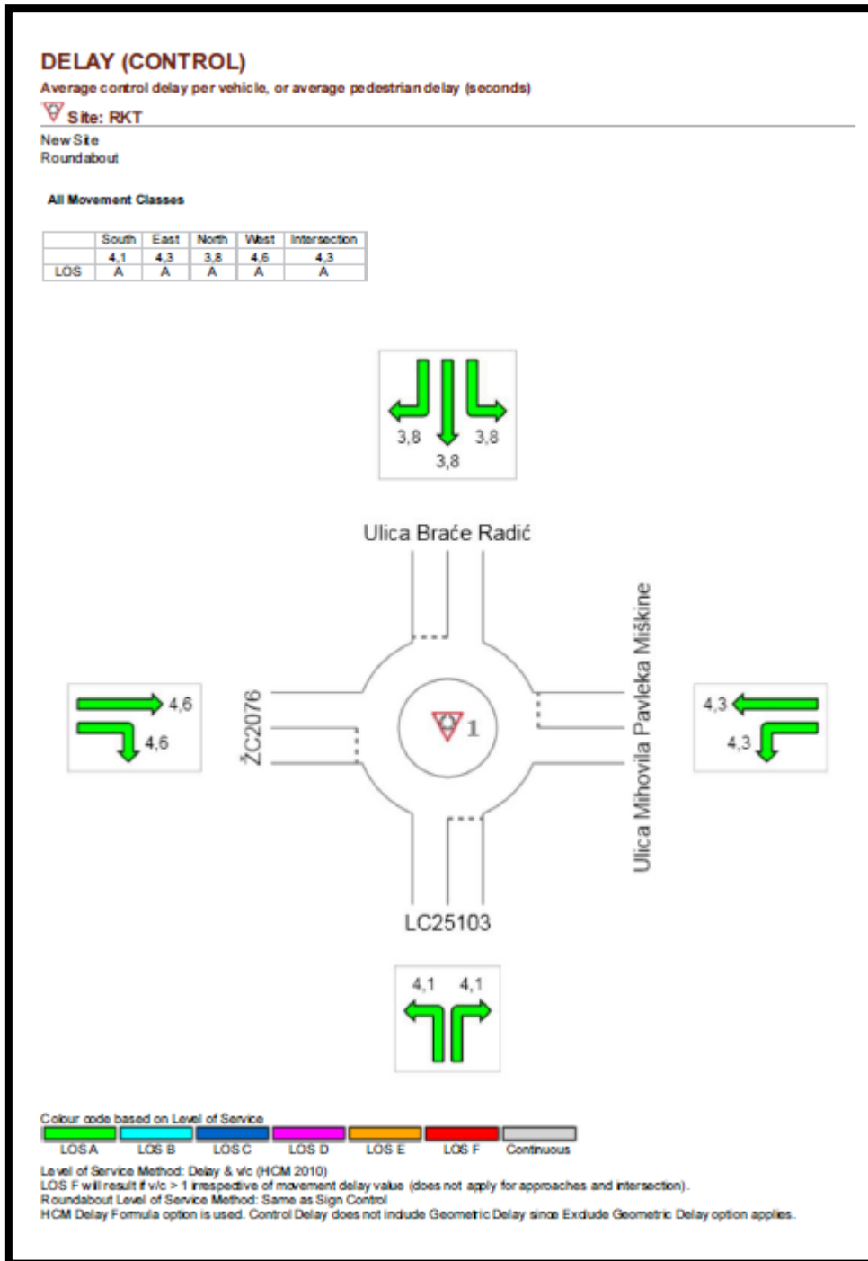
Slika 49. Prikaz rezultata prosječnog vremena kašnjenja dobivenih pomoću programskog alata SIDRA INTERSECTION
