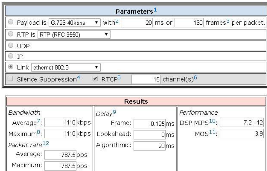
Slika 12. Rezultati analize G.726 bez detekcije tišine
