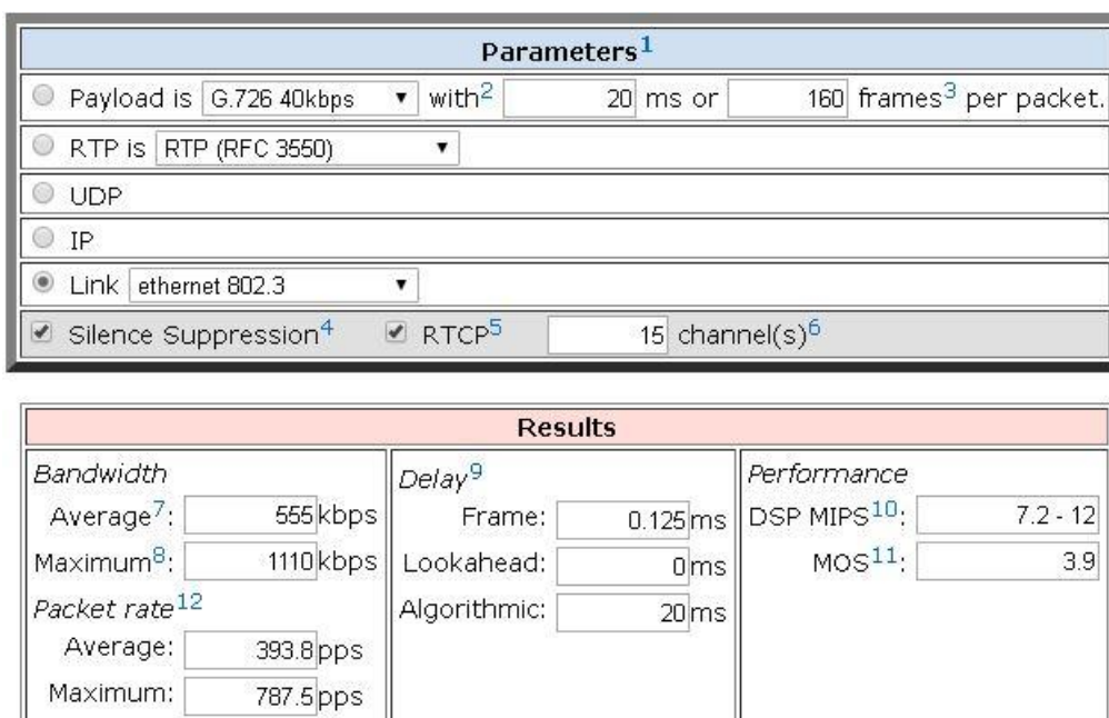
Slika 13. Rezultati analize G.726 s detekcijom tišine
