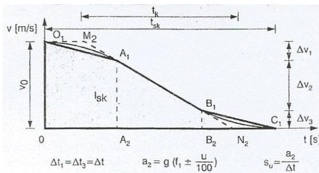
Slika 16. Dijagram brzine u ovisnosti o vremenu pri slobodnom koćenju [1]
