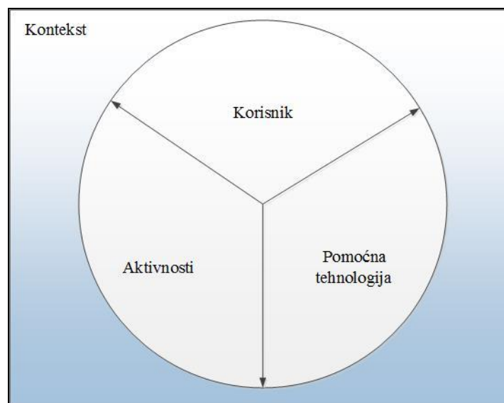
Slika 8. HAAT model, [3]
