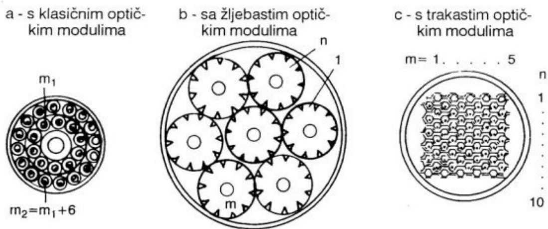
Slika 8. Formiranje jezgre optičkog kabela
