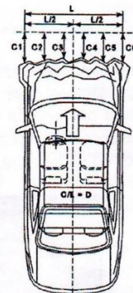
Slika 3.14. Prikaz podataka o veličini deformacije vozila, [11]
